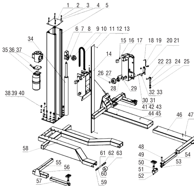
Рисунок 1 - Детализовка
