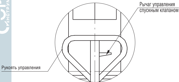
Рисунок 5 – Рукоять управления платформой
