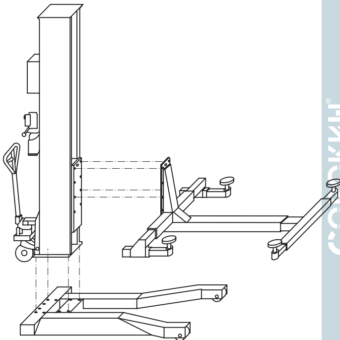
Рисунок 4 - Сборка каркаса
