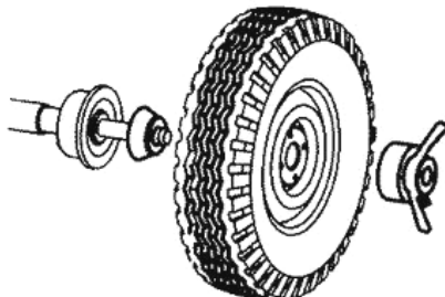
Рисунок 6.1 – Установка колеса
