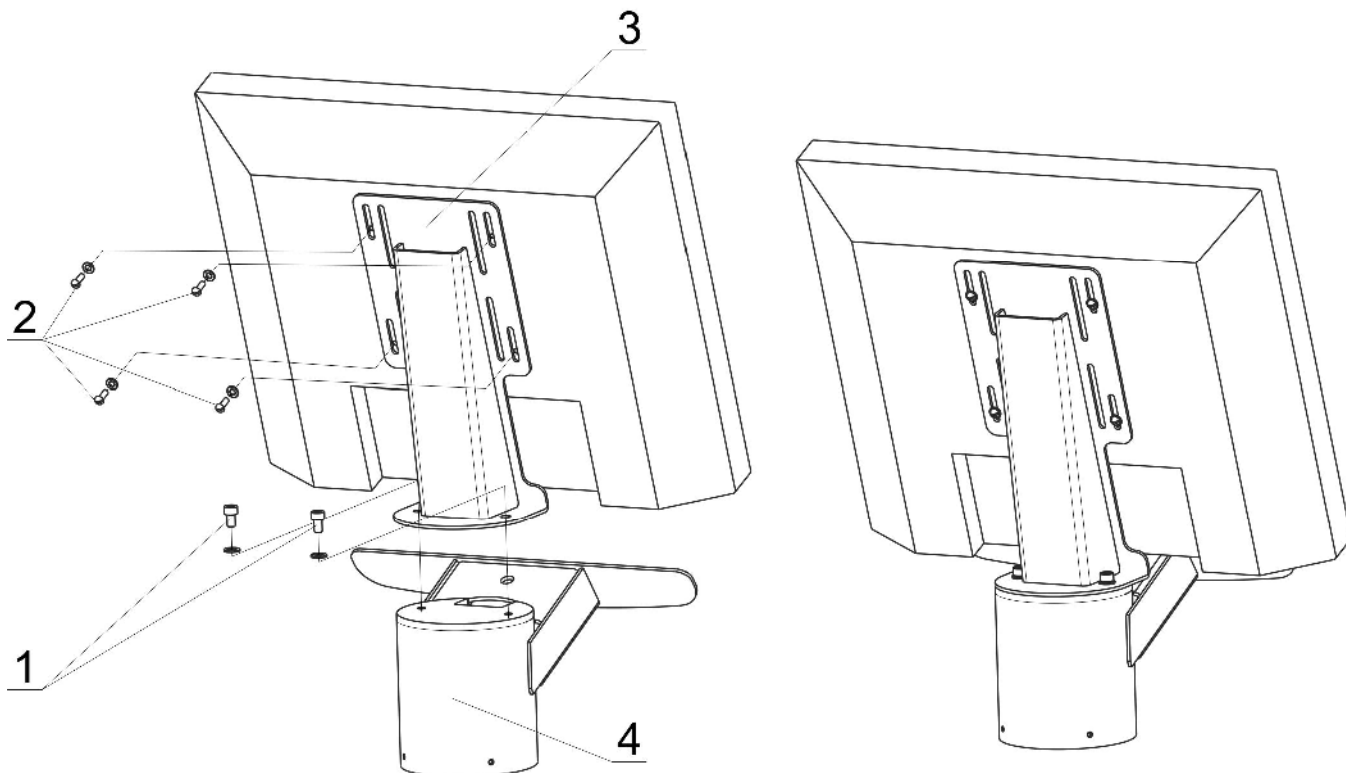
Рисунок 4.7 - Установка монитора
