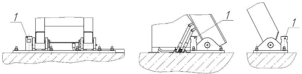
Рис. 4 Установка опор
