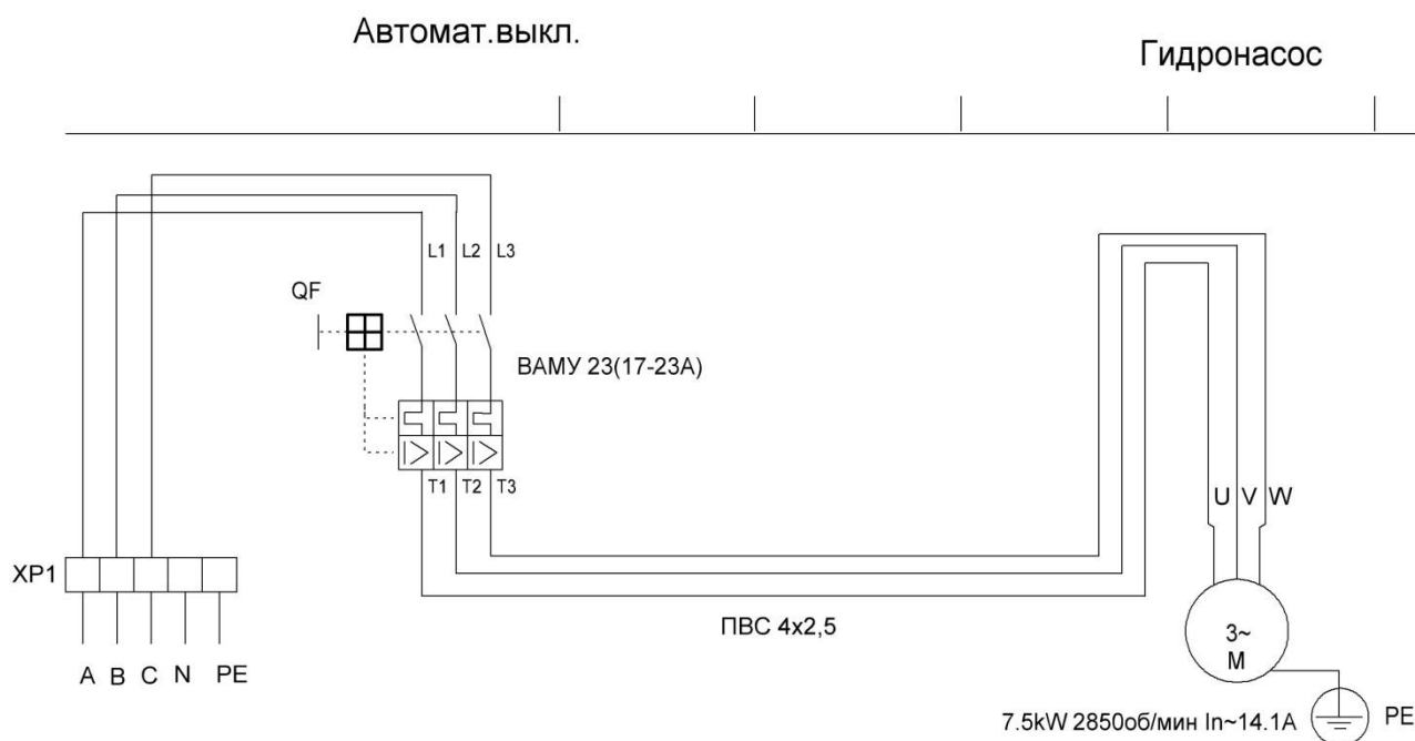
Рис. 2. Схема электрическая принципиальная 24Г272М1
