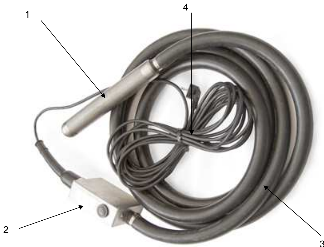
Рис.1 Внешний вид
