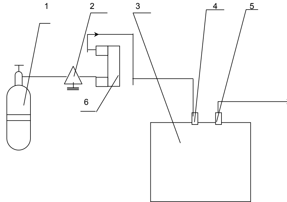
1 - Баллон ПГС; 2 - Вентиль тонкой регулировки; 3 – Прибор; 4 - Штуцер ВХОД ; 5 - Штуцер ВЫХОД; 6-Ротаметр
